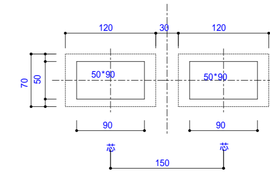
コンテンツ穴あけ寸法
